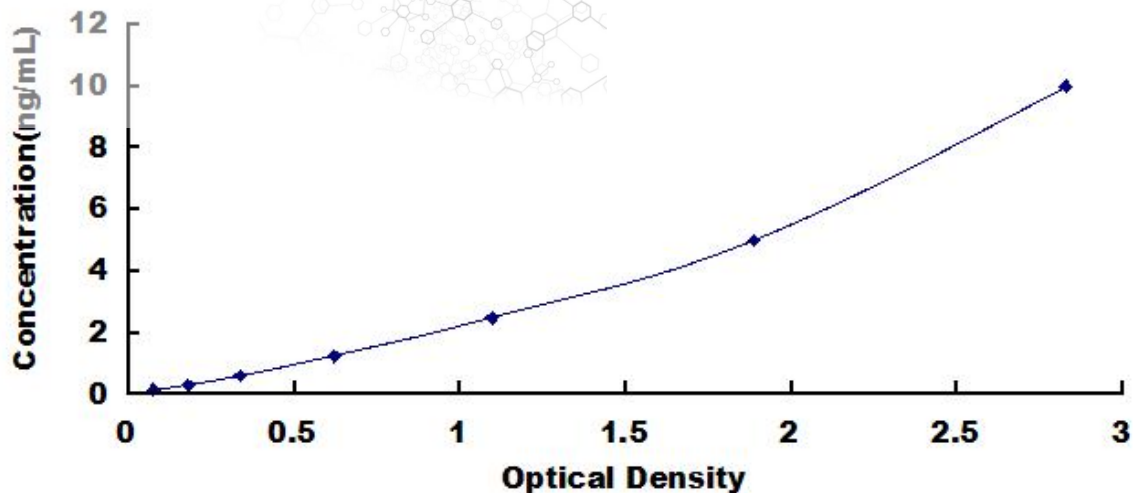
小鼠过氧化还原酶 1 (PRDX1) 检测试剂盒标准曲线
