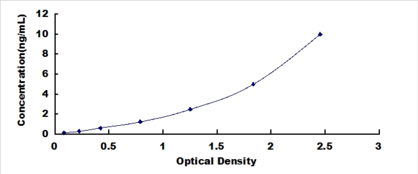
人调节激活正常 T-细胞表达分泌因子(RANTES)检测试剂盒标准曲线
